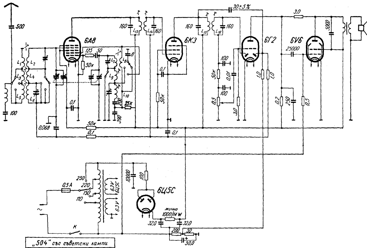
Фиг. 2.2.6. Схема на радиоприемника „Ворошидов“ тип 504 със съветски лампи
