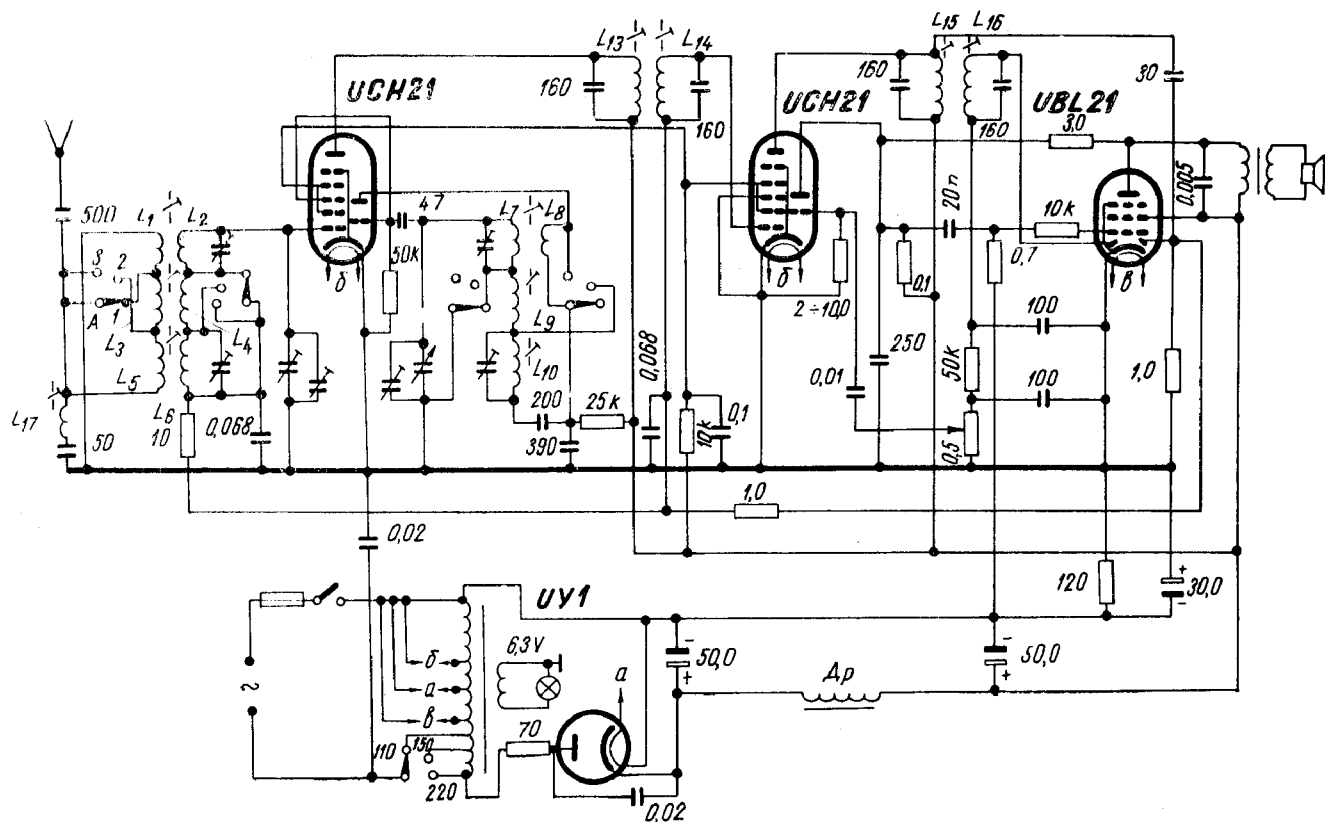
Фиг. 2.2.7. Схема на радиоприемника „Ворошилов“ тип 504 с лампи серия U 21
