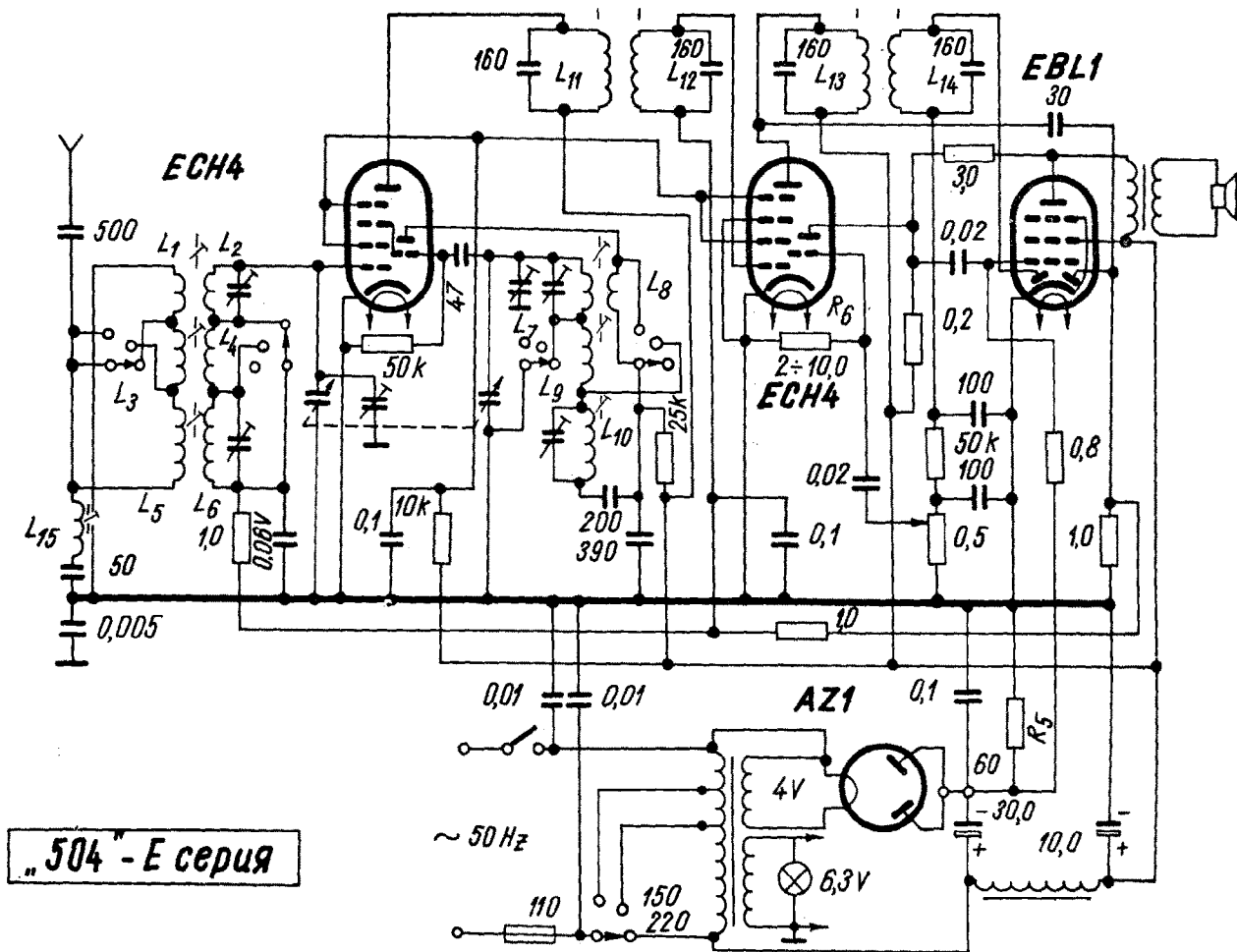
Фиг. 2.2.5. Схема на радиоприемника „Ворошилов“ тип 504 с лампи серия Е
