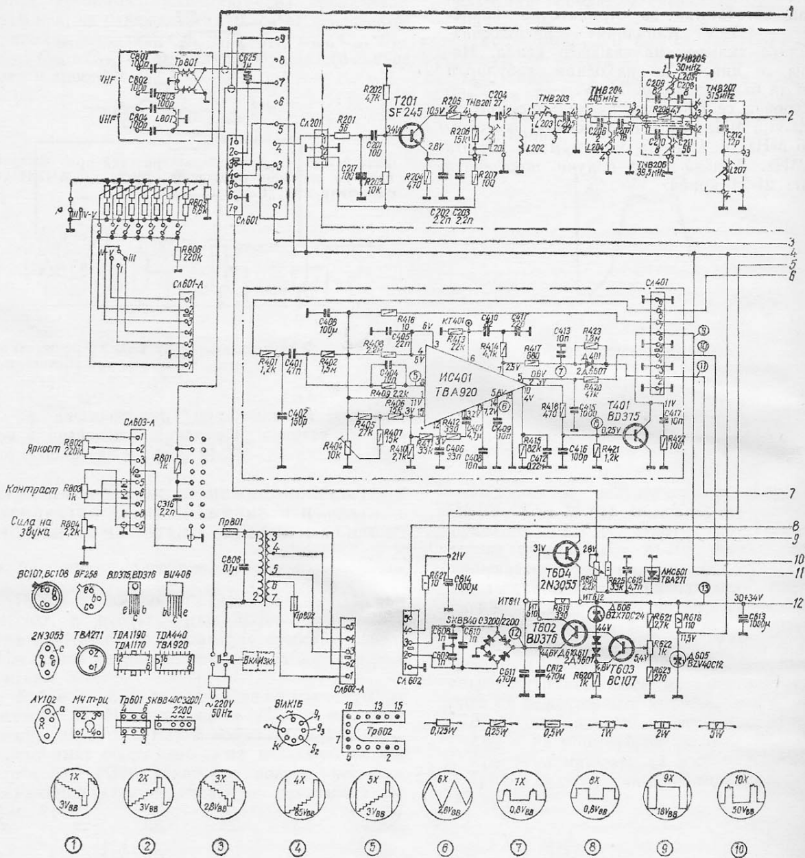
Приложение: Электрическая схема на телевизивизионния приемник „София 21“
