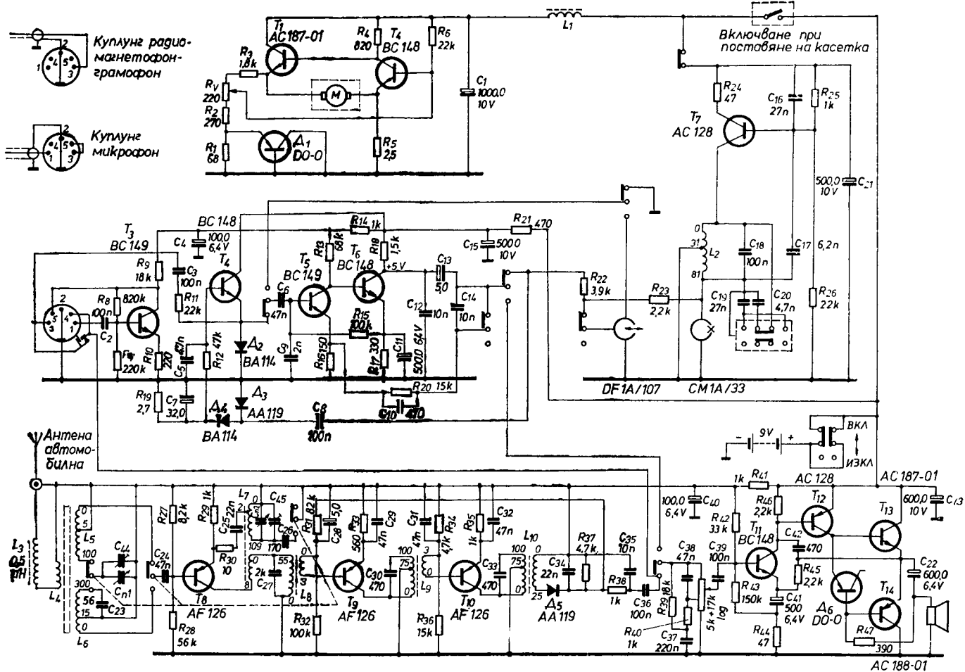
Фиг. 4.134. Принципна схема на радиомагнитофона „Октава“
