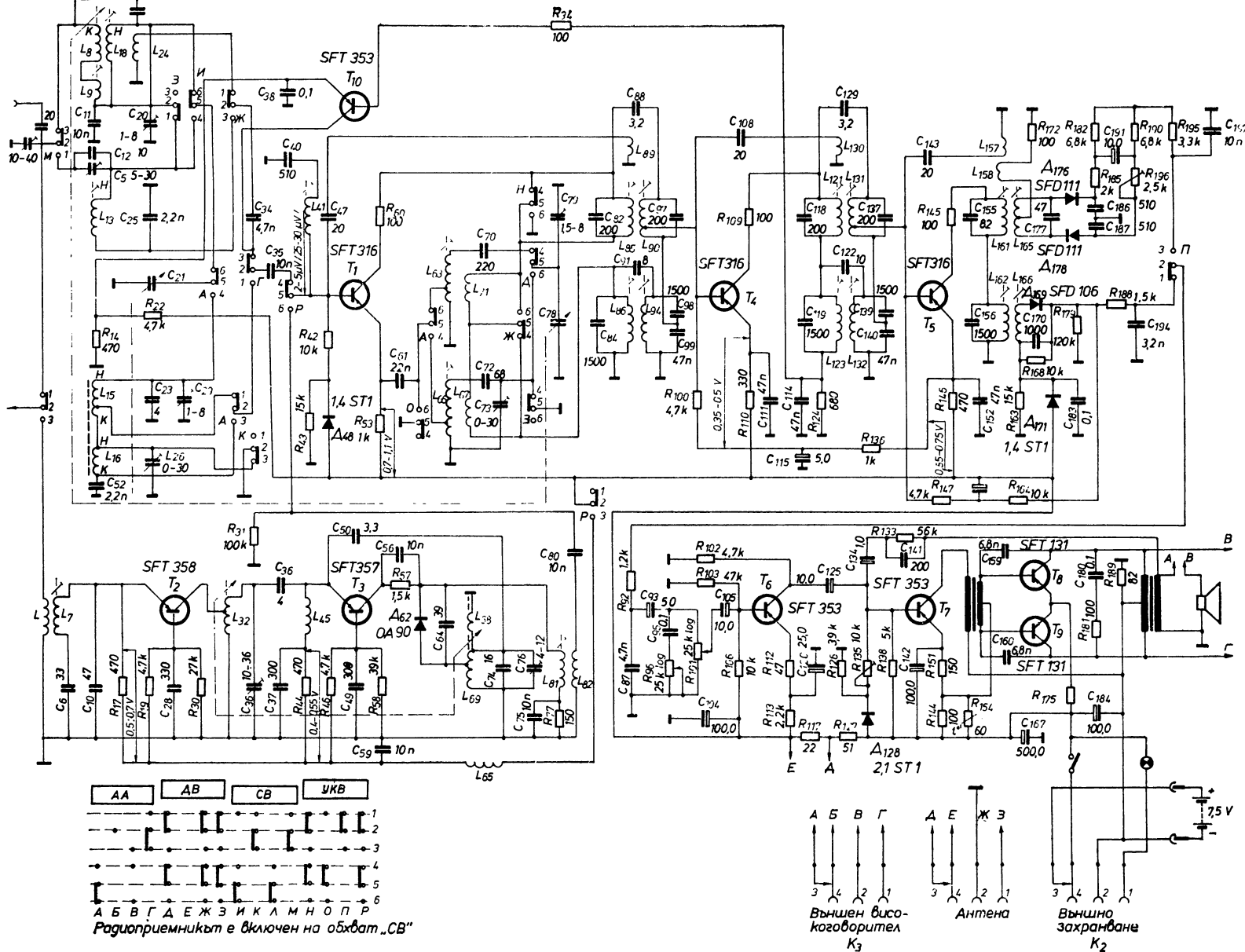
Фиг. 4.27. Принципно схема на радиоприемник „Универсал“
