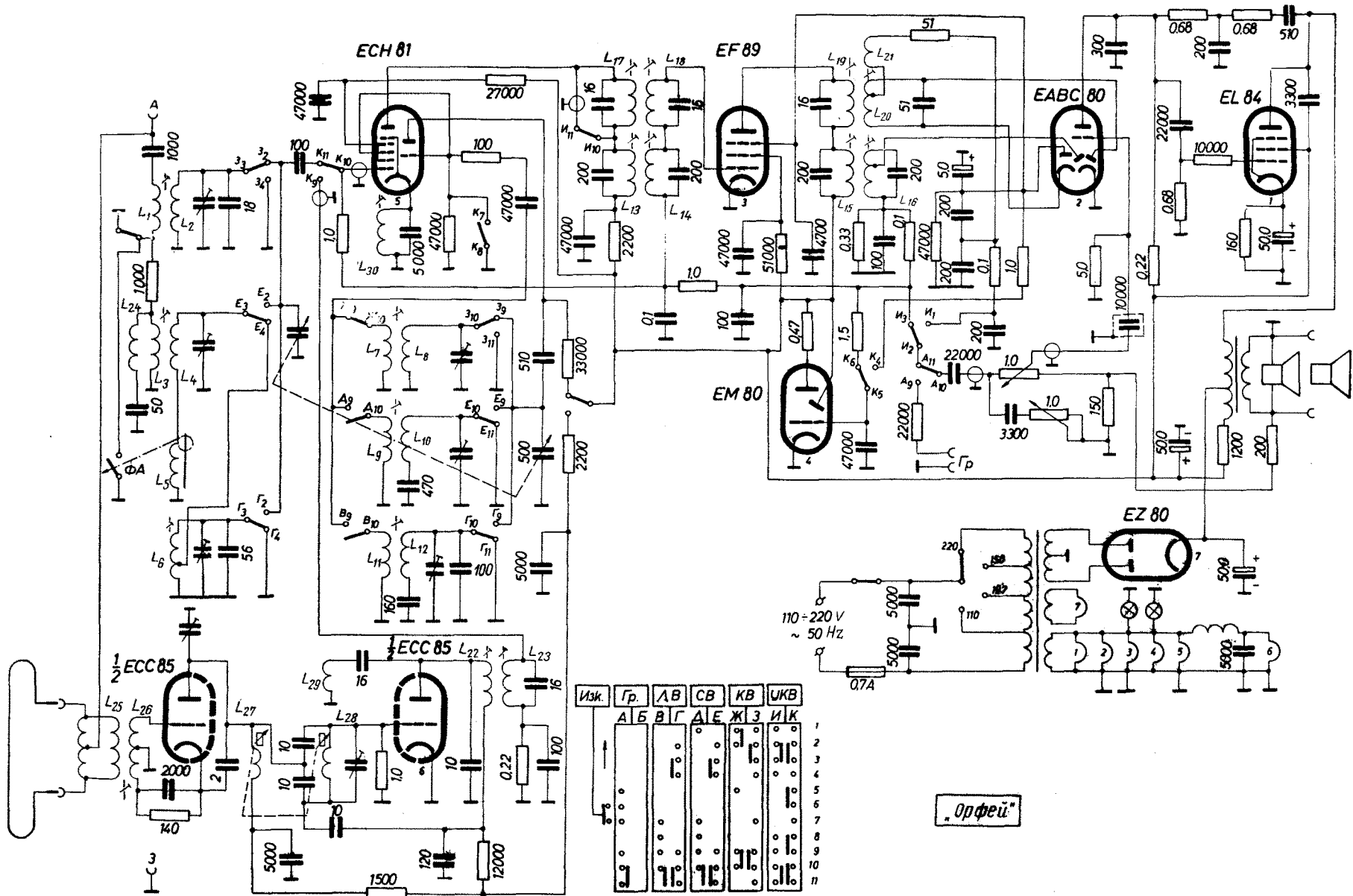
Фиг. 2.11.4. Схема на радиоприемника „Орфей“
