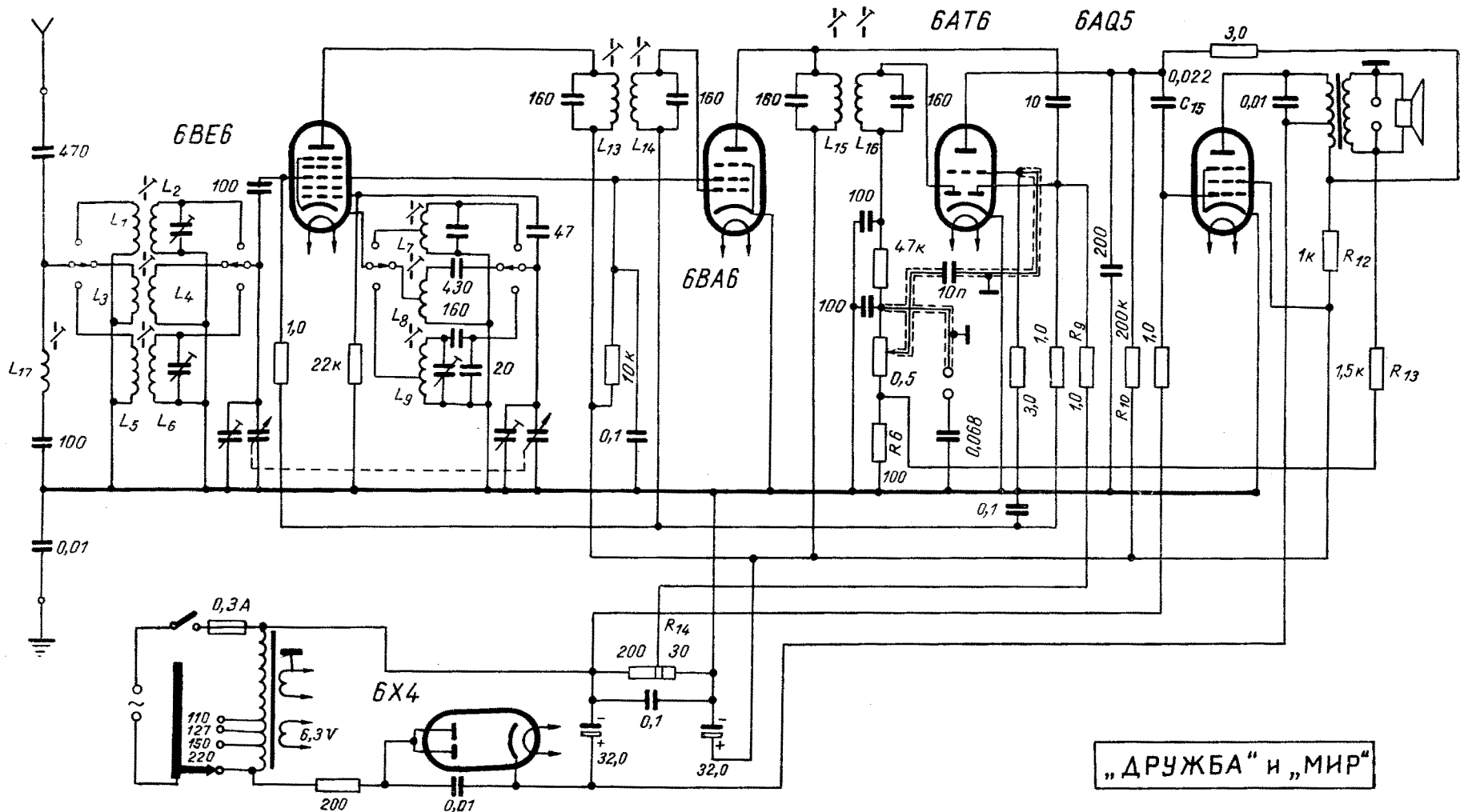
Фиг. 2.4.7. Схема на радиоприемниците „Дружба“ и „Мир“ с лампи от миниатюрната серия
