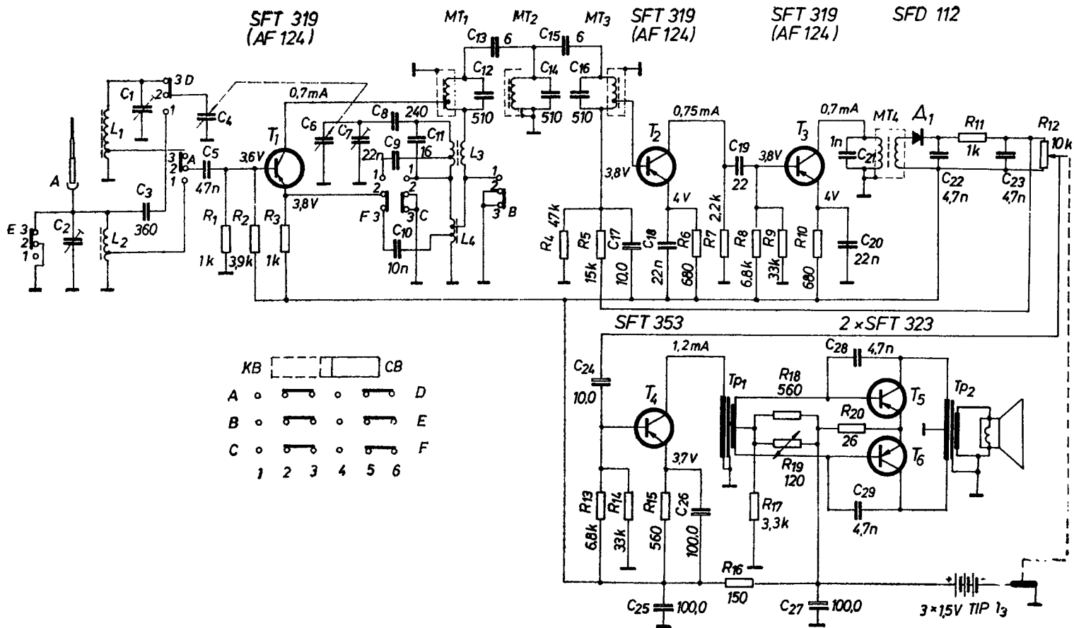
Фиг. 4.18. Принципна схема на радиоприемник „Ехо 2“
