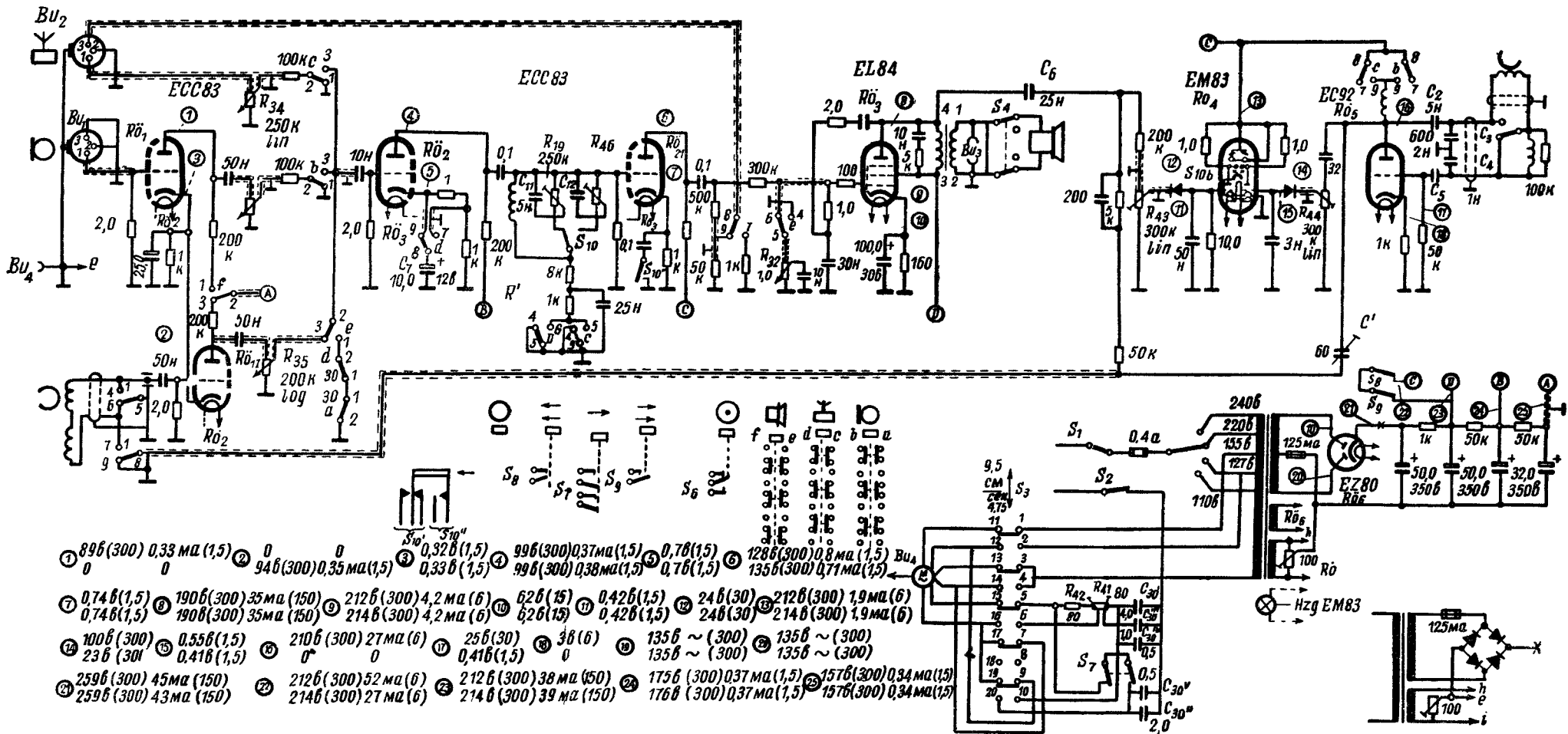
Фиг. 61. Схема на магнитофон KB-100
